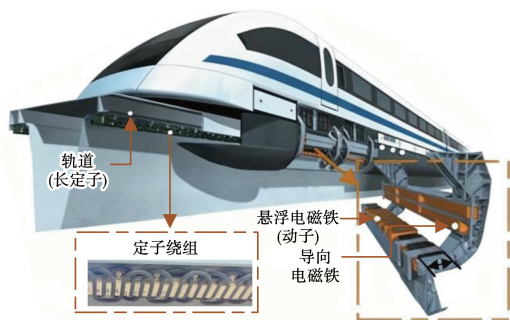
图1 高速磁悬浮列车的结构图
