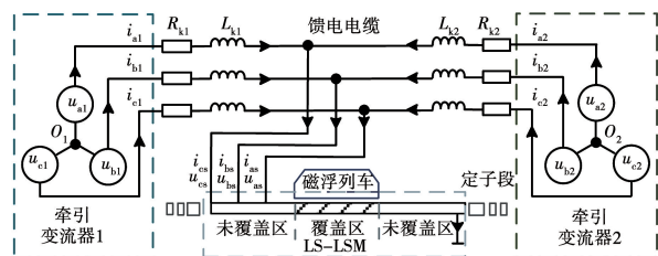
图2 高速磁悬浮列车在双端供电模式牵引供电系统原理图
