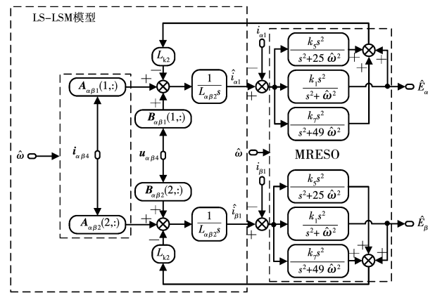
图8 MRESO 的结构图
