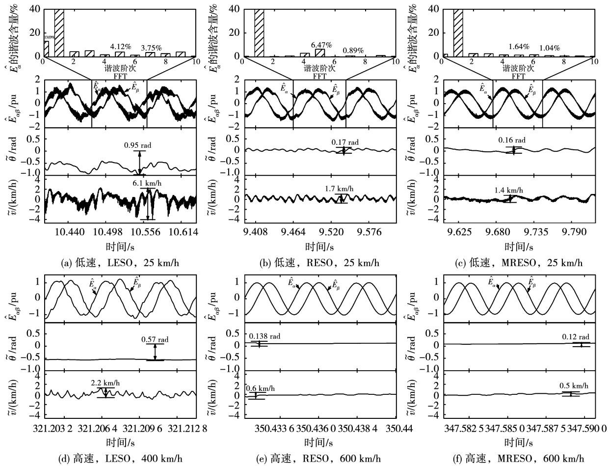
图 13 不同反电动势观测算法的实验结果对比
