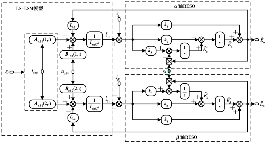
图5 RESO 的结构图
