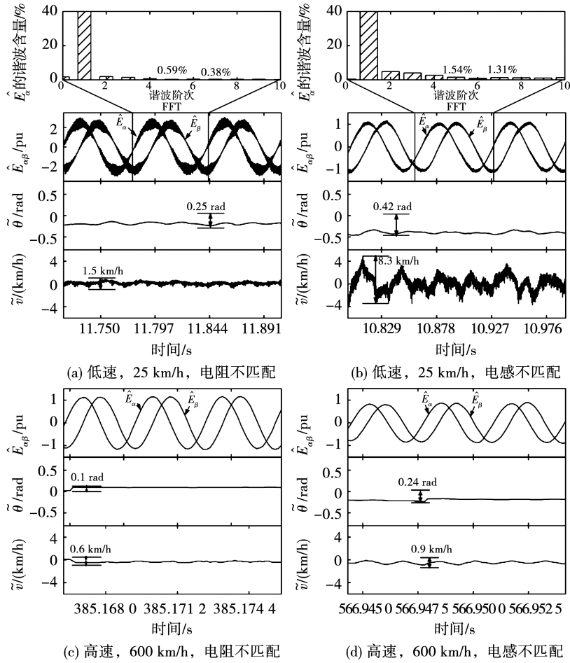
图 14 参数不匹配时 MRESO 的实验结果
