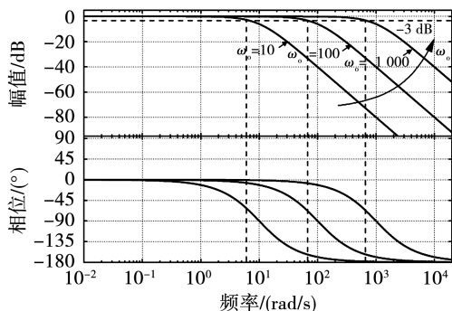
图3 带宽变化时 LESO 的 Bode 图
