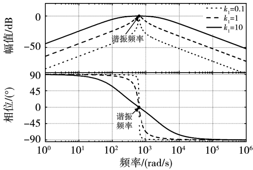
图7 仅保留参数 k_1 时 RESO 的 Bode 图
