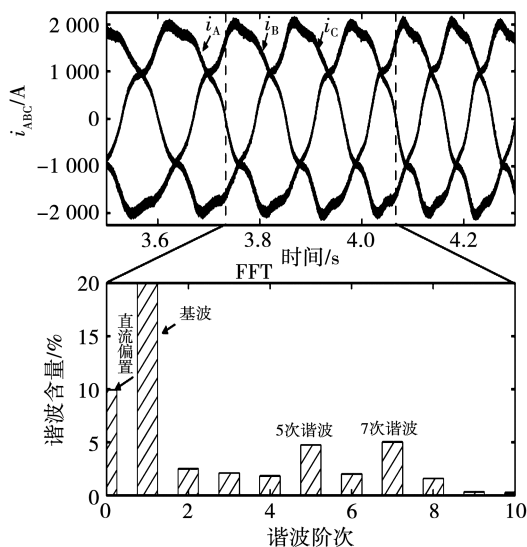
图4 三相电流波形及其 FFT 分析
