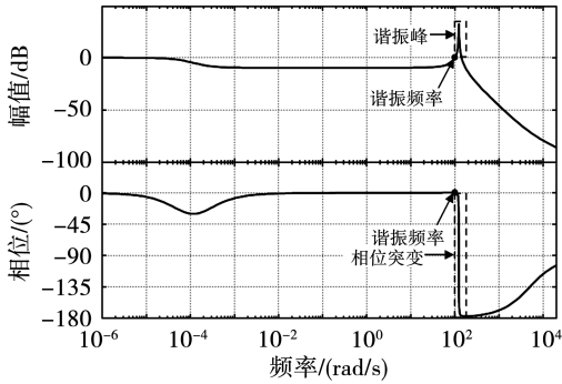
图6 RESO 的 Bode 图
