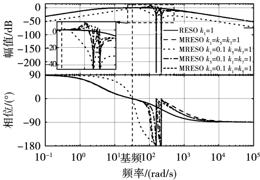
图 9 RESO 和 MRESO 的 Bode 图
